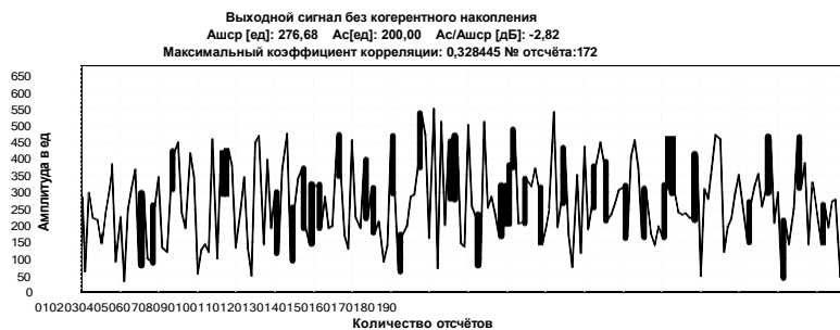
Рисунок 3 – Вид сигнала при отношении сигнал/шум - 2,82 дБ
