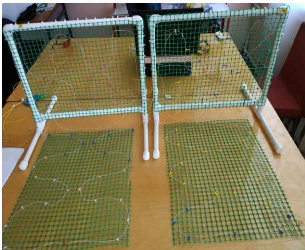
Рисунок 3 – Опытный образец четырех канальной волоконно-оптической системы охраны
